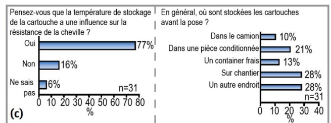
Figure 13: De nombreux poseurs ne sont pas conscients de l'influence des facteurs importants sur la capacité d'ancrage:
