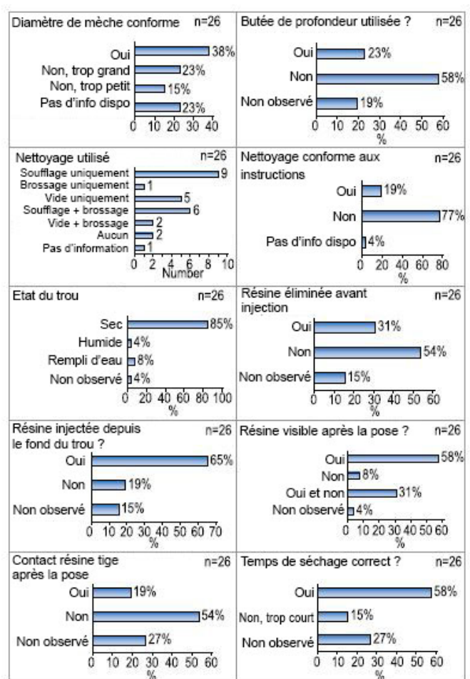
Figure 2: Résultats de l'étude terrain sur la pose d'ancrages chimiques. (n= nombre d'applications observées)
