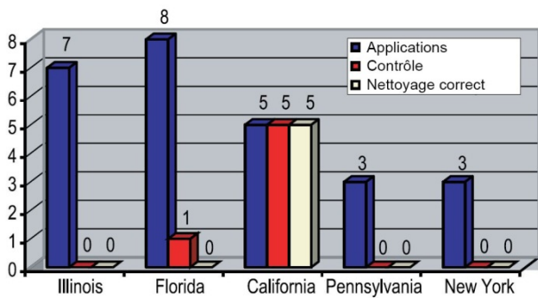
Figure 10: Influence des contrôles sur la pose des ancrages. Le nettoyage correct des trous n'a été observé qu'en Californie, un état avec une longue expérience datant de l'UBC.
