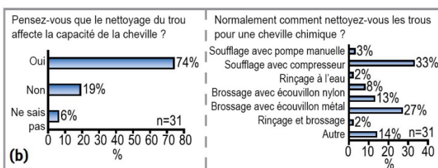
Figure 13: De nombreux poseurs ne sont pas conscients de l'influence des facteurs importants sur la capacité d'ancrage:
